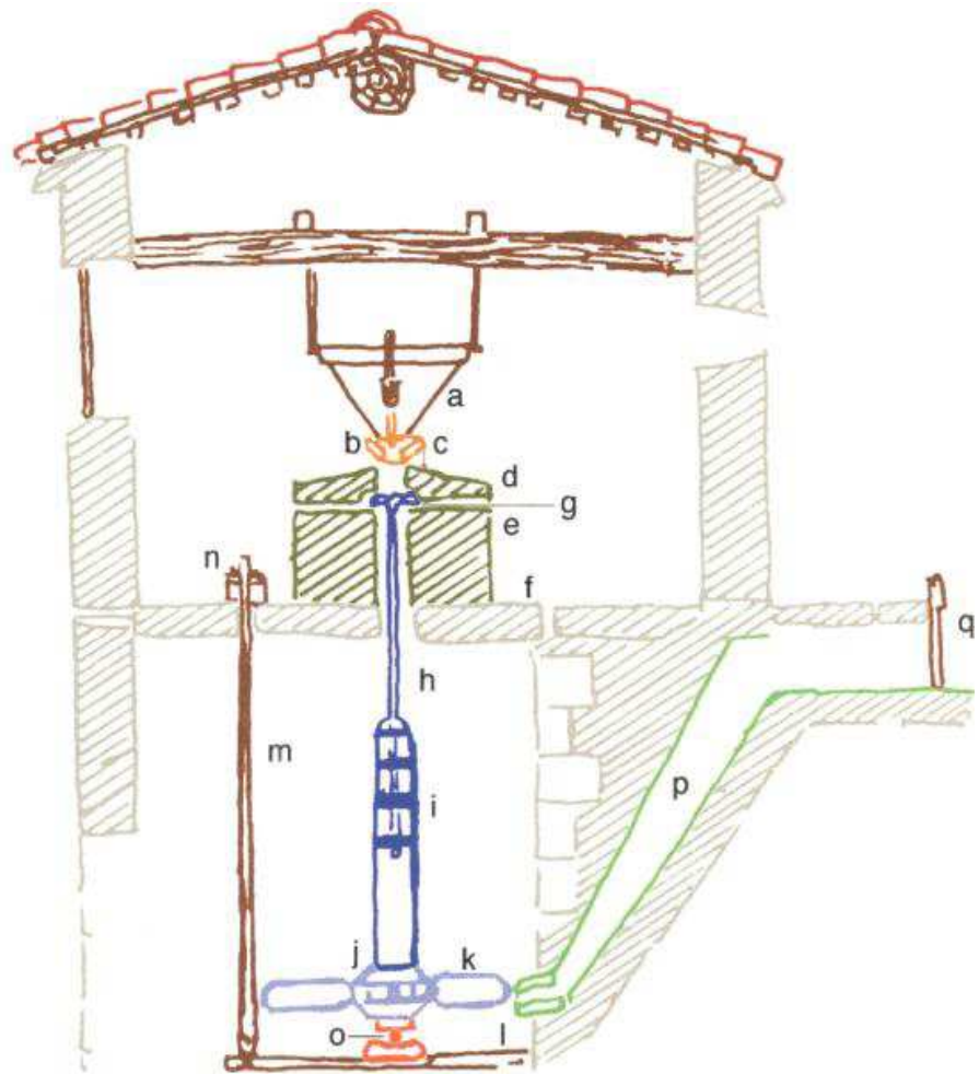
Corte esquemático de um moinho de rodízio
